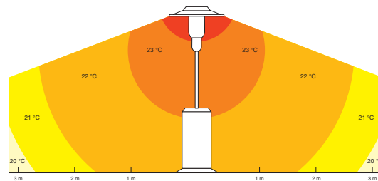
TEPLOTNÍ SCHÉMA při 10 °C venkovní teploty
