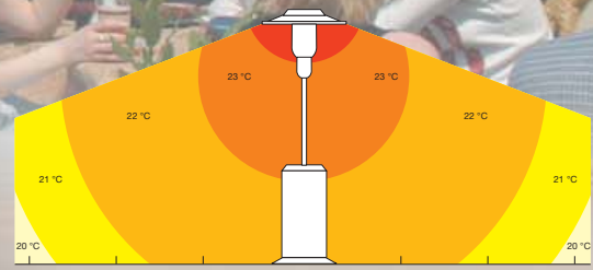
TEPLTNÍ SCHÉMA při 10 °C venkovní teploty
